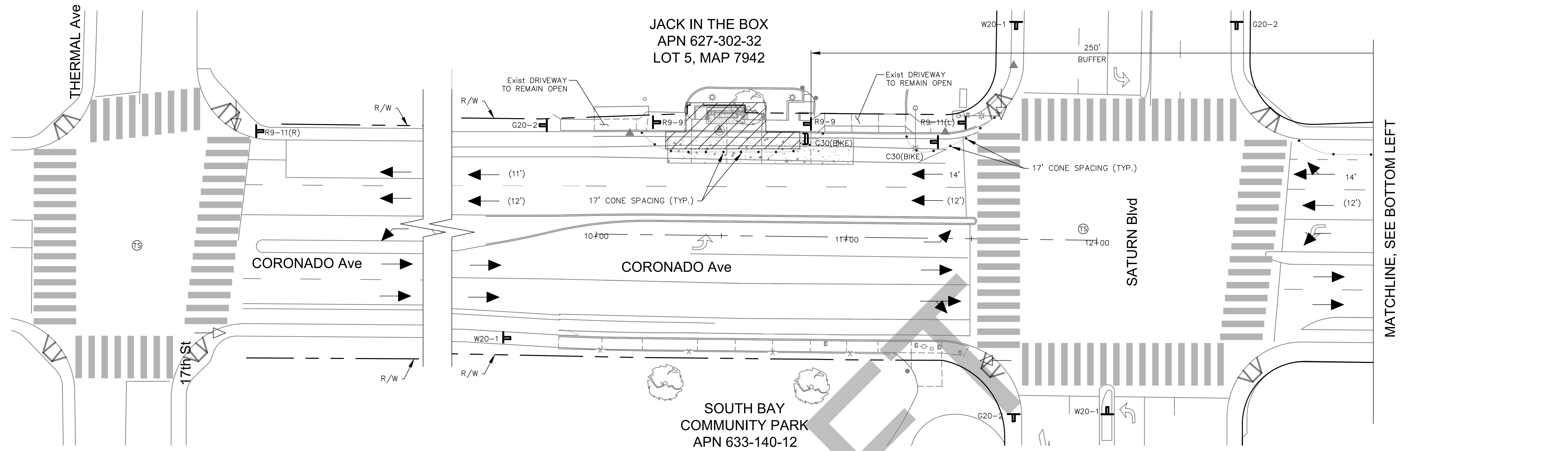
PLAN SCALE: 1" = 20'
